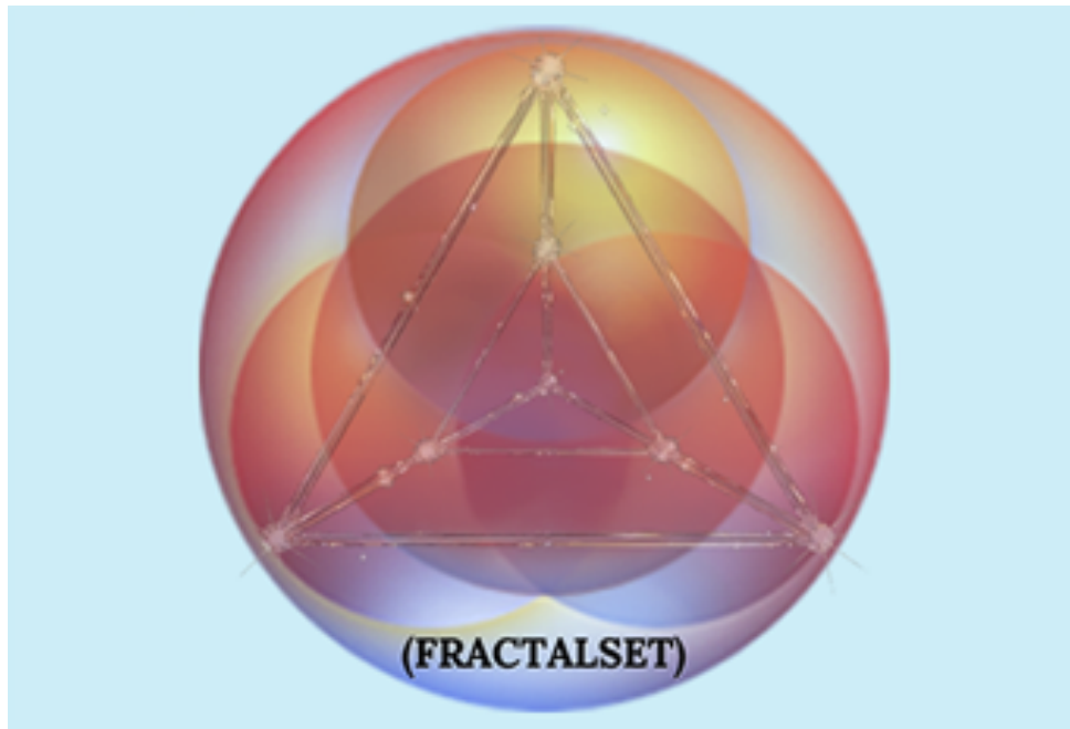
Figura 04: Detalhe da Estrutura tetraédrica do Fractalset: Arquitetura Quadriuna da Manifestação – Elaboração de Júlio Torres
