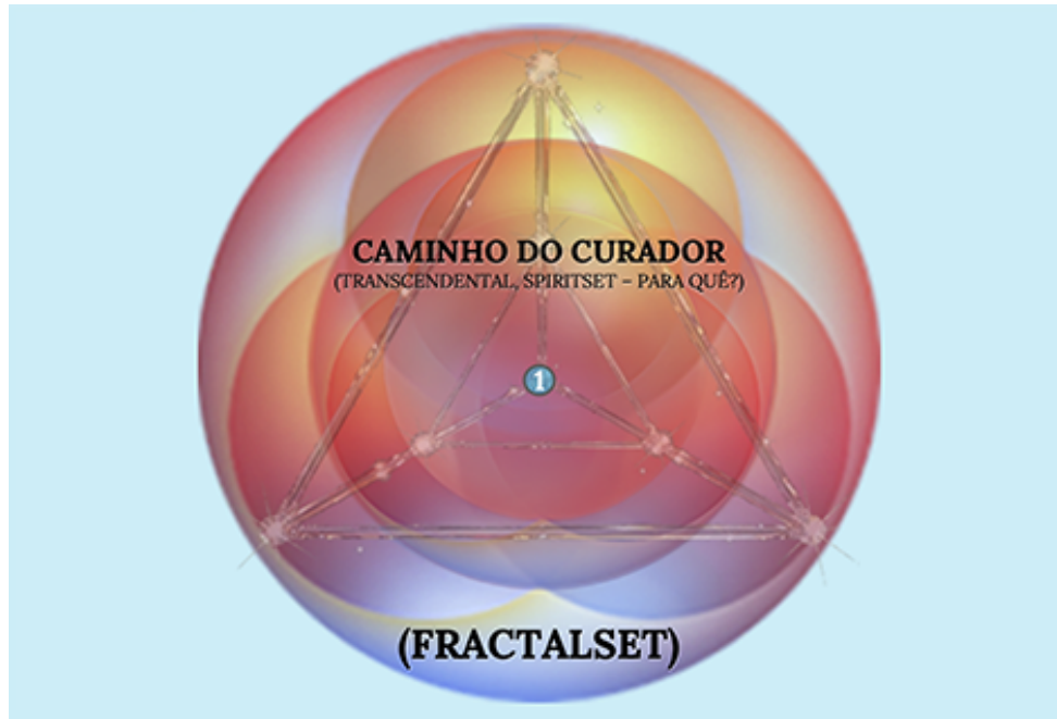
Figura 05: Detalhe da Estrutura Fractal do Caminho do Curador na Arquitetura Quadriuna da Manifestação – Elaboração: Prof. Júlio Torres
