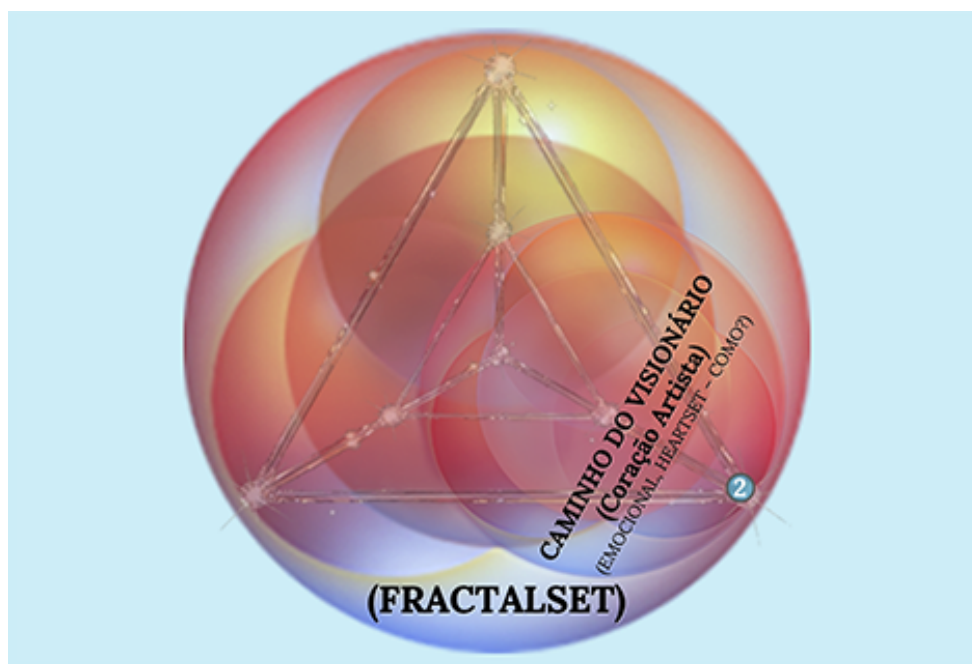
Figura 06: Detalhe da Estrutura Fractal do Caminho do Visionário (Coração Artista) na Arquitetura Quadriuna da Manifestação – Elaboração: Prof. Júlio Torres
