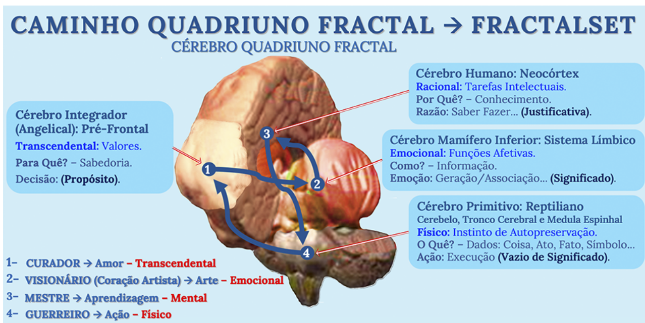
Figura 01: Fractalset: Caminho Quadriuno Fractal e Cérebro Quadriuno Fractal – as quatro Dimensões do Ser Integral e sua perguntas constitutivas – Elaboração de Júlio Torres
