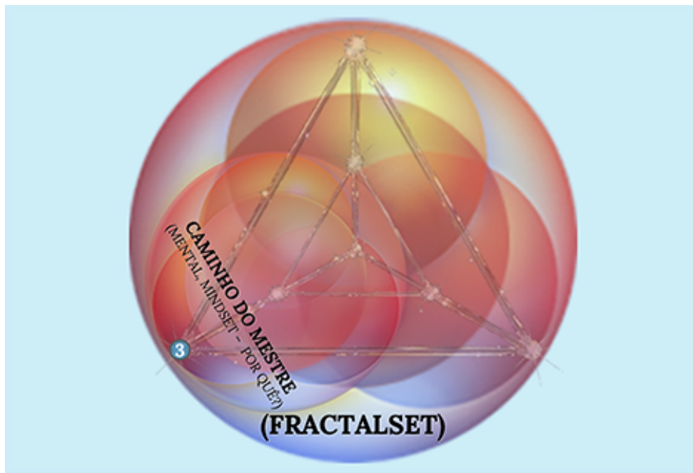
Figura 07: Detalhe da Estrutura Fractal do Caminho do Mestre na Arquitetura Quadriuna da Manifestação – Elaboração: Prof. Júlio Torres
