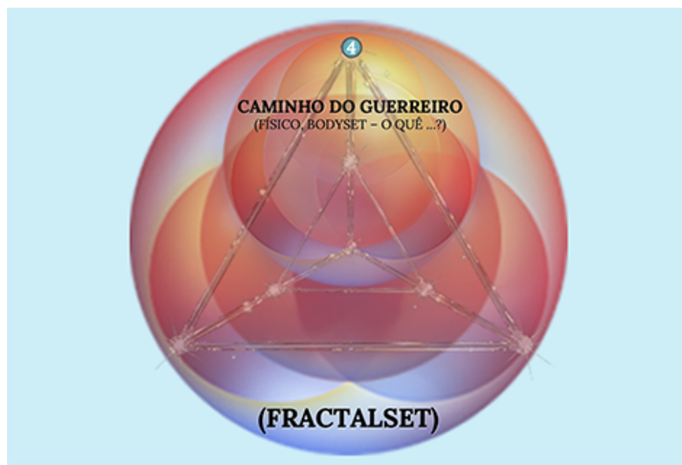
Figura 08: Detalhe da Estrutura Fractal do Caminho do Guerreiro na Arquitetura Quadriuna da Manifestação – Elaboração: Prof. Júlio Torres
