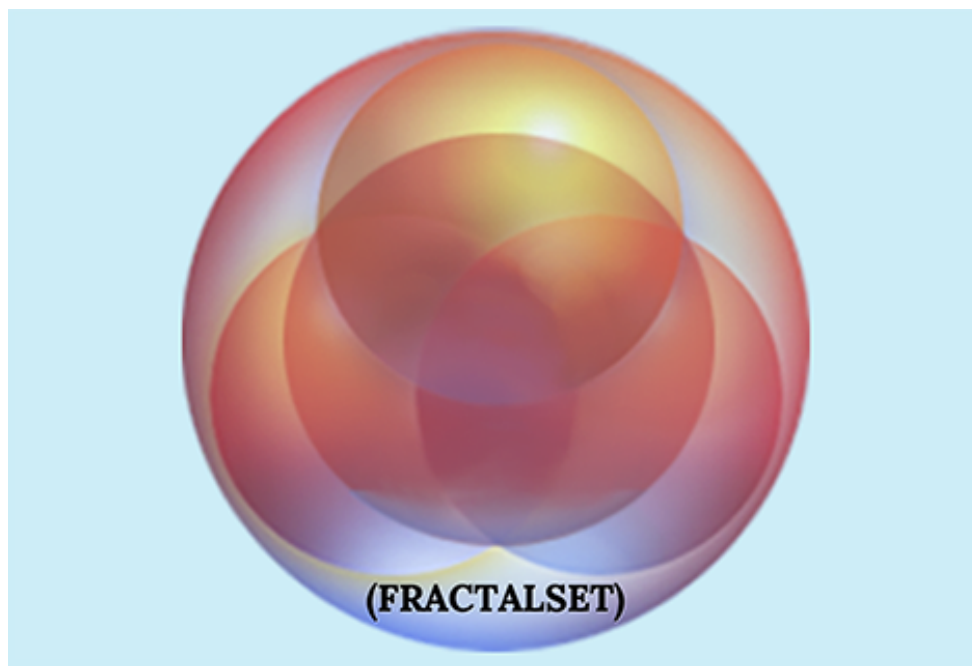
Figura 03: Detalhe da Representação Fractal do Fractalset: Arquitetura Quadriuna da Manifestação – Elaboração de Júlio Torres
